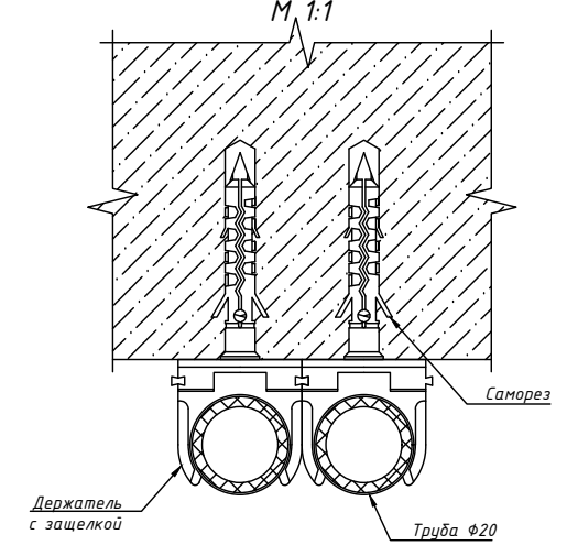
Эскиз крепления кабельной трассы М 1:1
